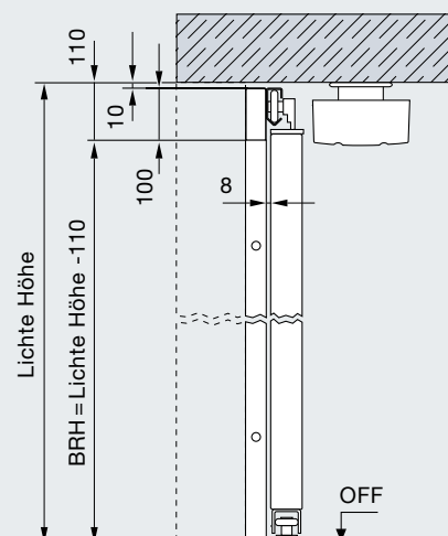
Vertikalschnitt
